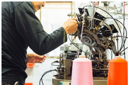
筒型の編み機に糸をセット
